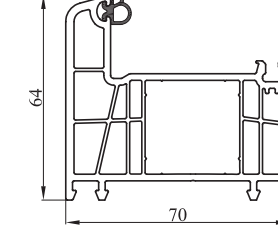
Ościeżnica okienna i balkonowa nr: 7110-01 profil biały z uszczelką szarą nr: 7110-02 profil biały z uszczelką czarną
