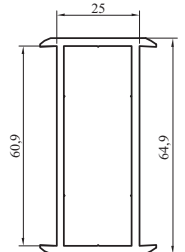
Łącznik statyczny nr: 6053
