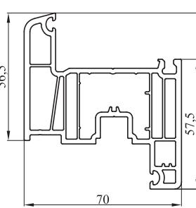
Skrzydło okienne i balkonowe nr: 7120-01 profil biały z uszczelką szarą nr: 7120-02 profil biały z uszczelką czarną
