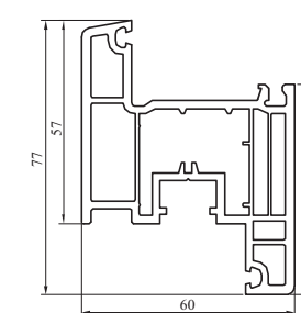
Skrzydło okienne i balkonowe półzłocowane nr: 6021
