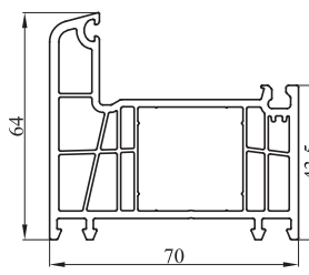
Ościeżnica okienna i balkonowa nr: 7110-01 profil biały z uszczelką szarą nr: 7110-02 profil biały z uszczelką czarną
