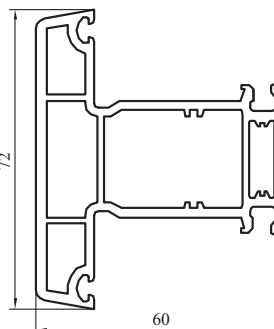
Słupek stały nr: 6030
