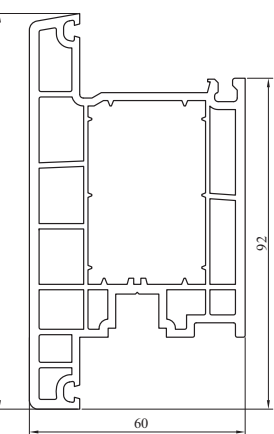
Skrzydło drzwiowe T nr: 6025
