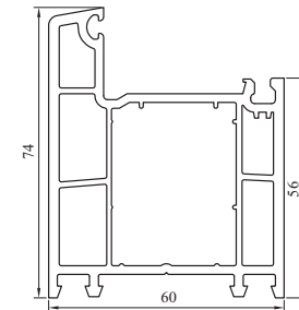
Skrzydło okienne i balkonowe nr: 6020
