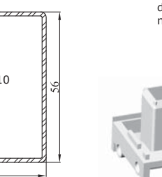
Łącznik progu 7018 z ramą 7012 nr: 90-327-00
