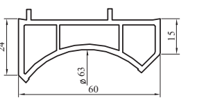
Łącznik rurowy - część zewnętrzna nr: 6055
