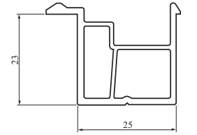
Listwa podokienna nr: 6057
