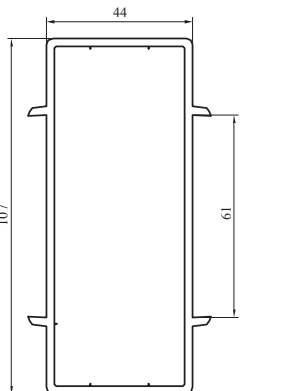
Łącznik statyczny - fasadowy nr: 6056
