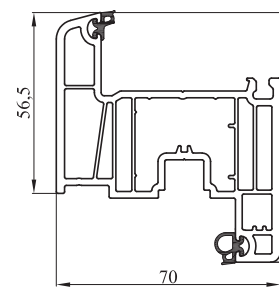
Skrzydło okienne balkonowe poszerzone nr: 7126-00 profil biały
