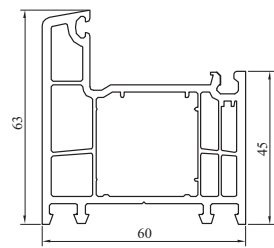
Ościeżnica drzwiowa nr: 6012
