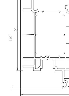
Skrzydło drzwiowe Z nr: 6024
