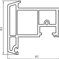
Słupek ruchomy nr: 6032
